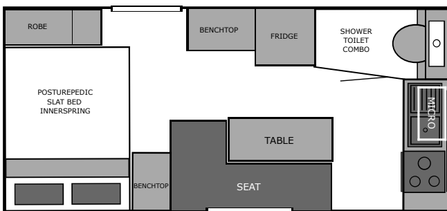
15'X7'6"-2 SPRINTER
