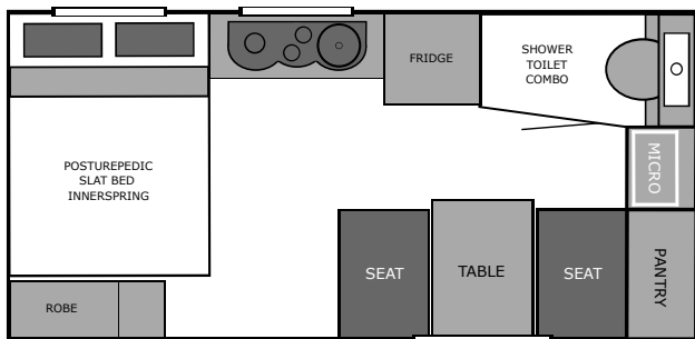
14'6"X7'6"-1 SPRINTER
